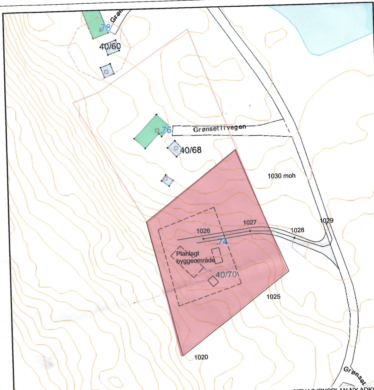
SITUASJONSPPLAN NY ADKOMSTVEG 1:1000
