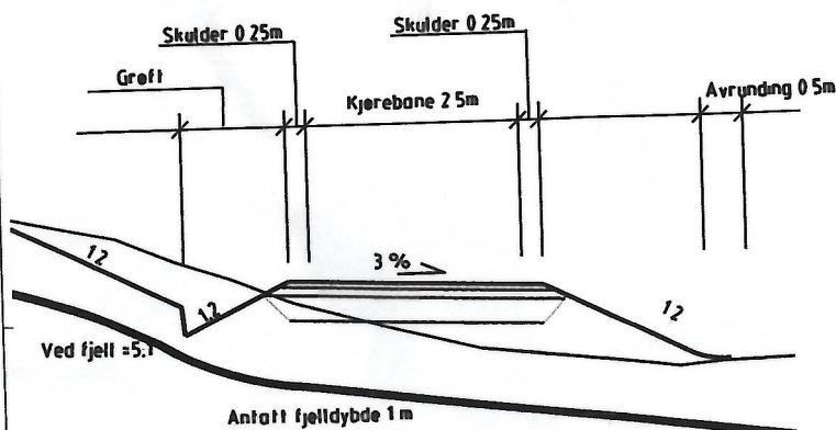
Normalprofil veg ved total vegbredde 3 m
