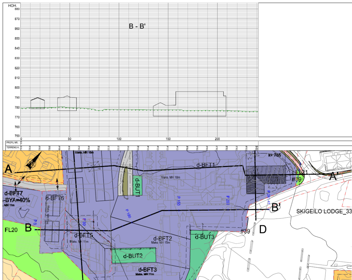
Figur 29: Snitt B-B'.
