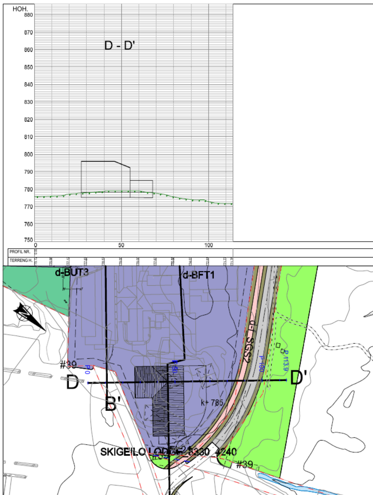
Figur 31: Snitt D-D'.
