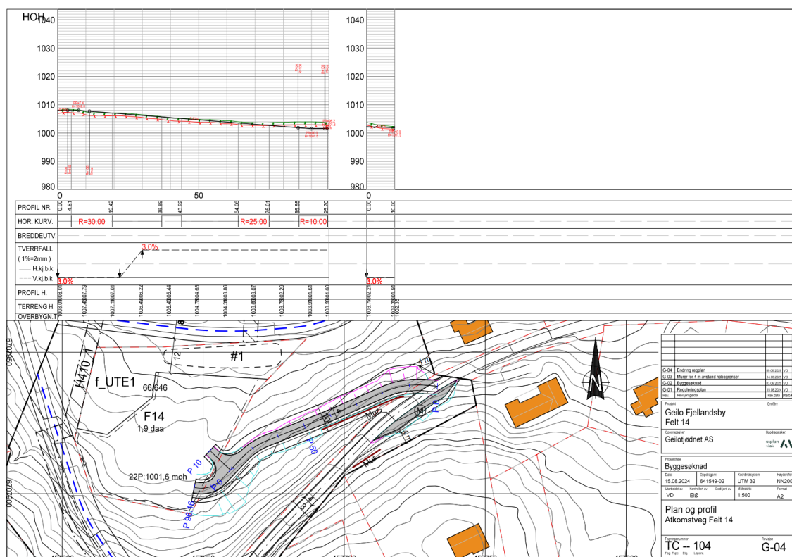
Figur 9: Plan og profil ny veg.
